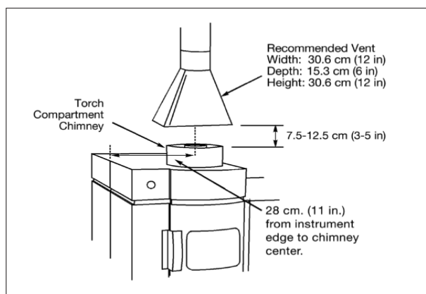
Figura 3. Campana de extracción de gases para el equipo ICP.
